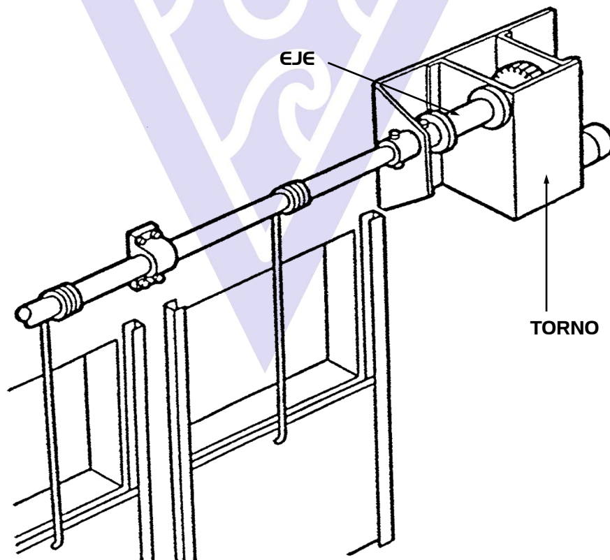
Sistema de control de transmisión de eje a tubo.
