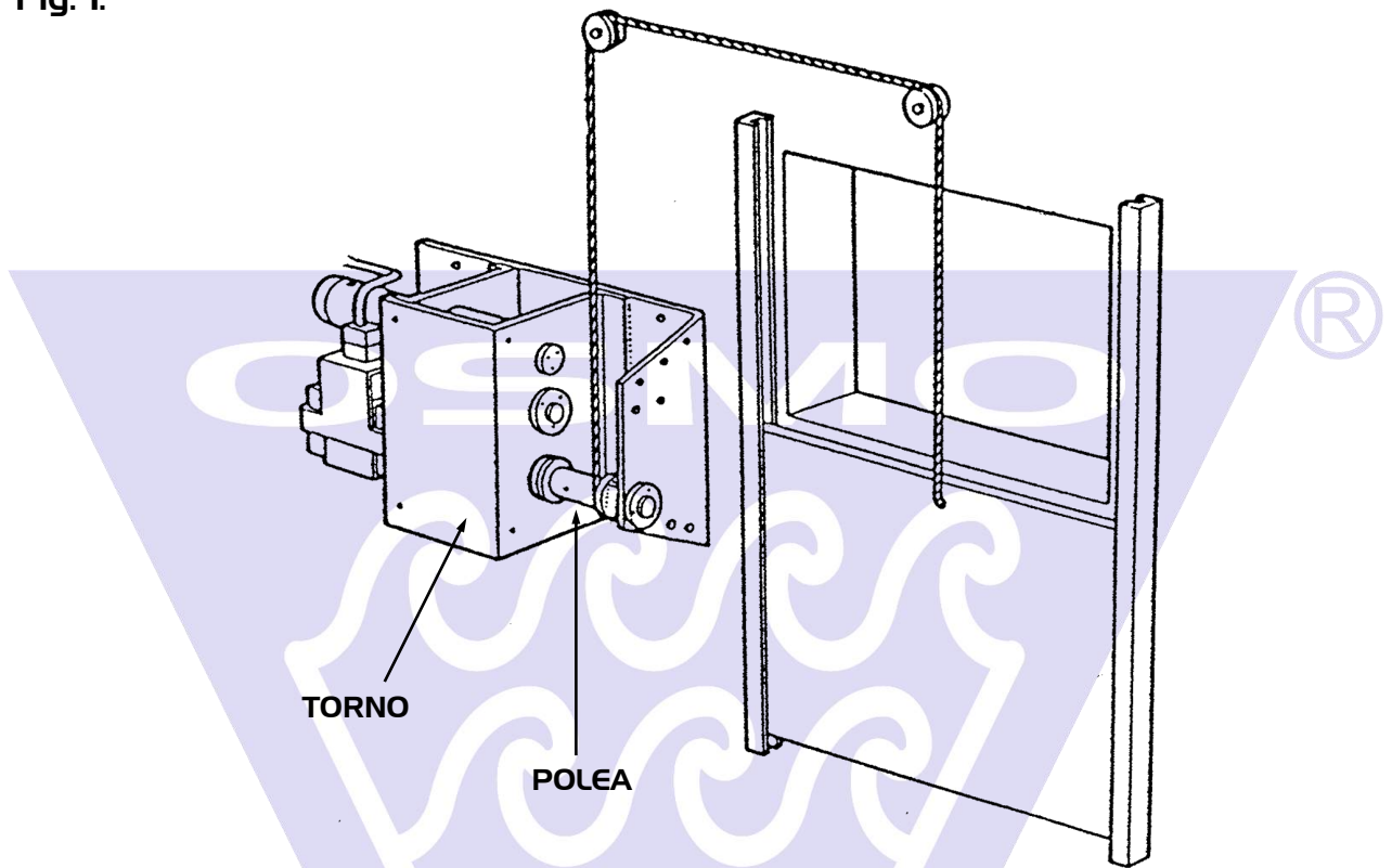
Sistema de control de ventanas de transmisión de sirga por polea.
